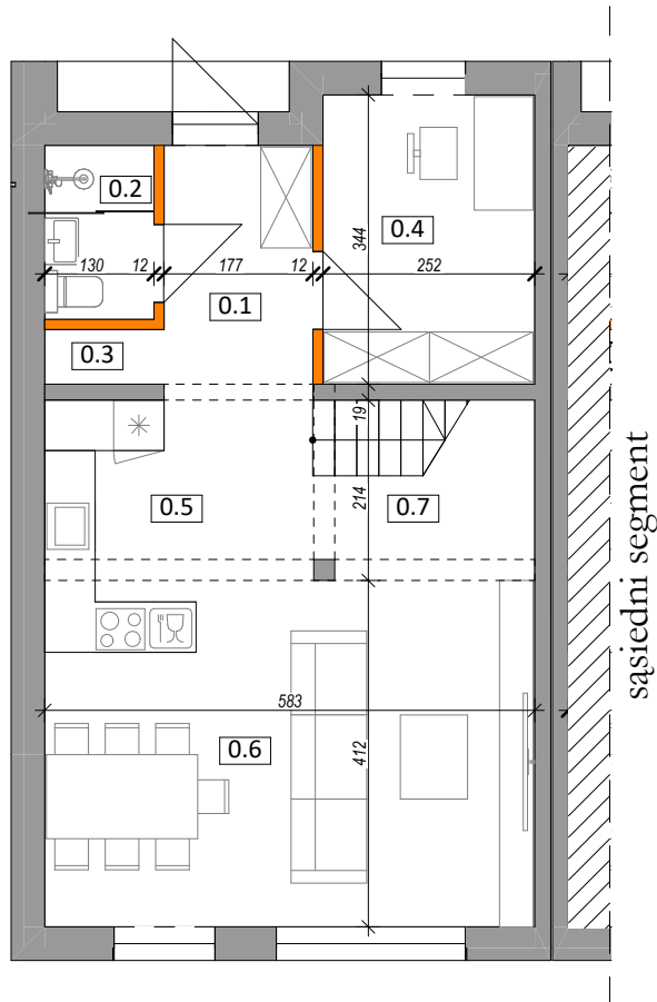
RZUT PARTERU
