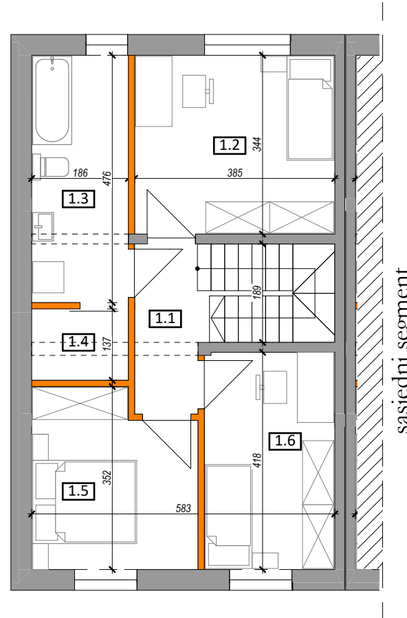
RZUT PIĘTRA
