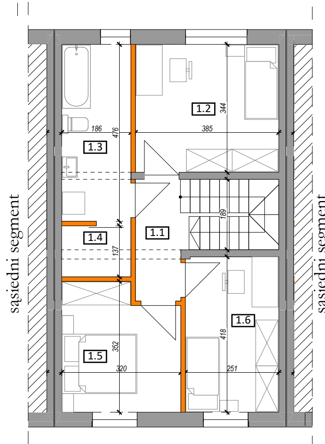
RZUT PIĘTRA
