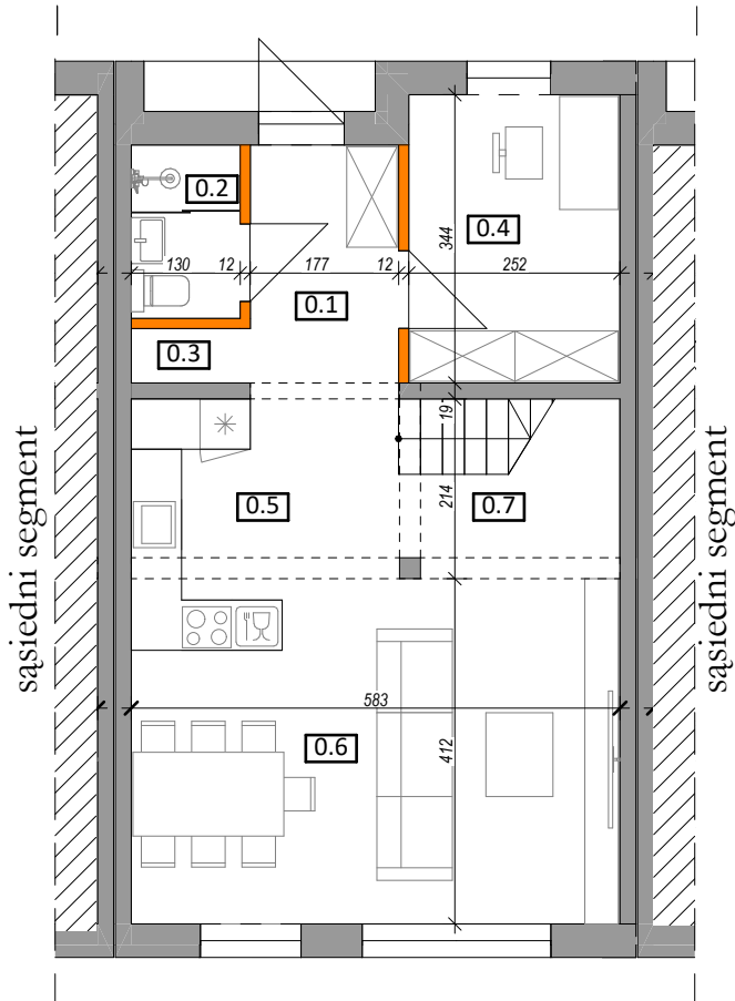
RZUT PARTERU
